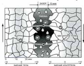
рис. 1: Конструктивное биение подшипников второго класса точности диаметром 40 мм. При трении металлических поверхностей возникают электромагнитные поля, которые захватывают атомарный водород (продукт деструкции масла) и направляют его в подложку металла.
