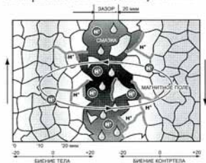
рис. 2: С ростом зазоров биение увеличивается пропорционально (в 2 раза). Атомарный водород накапливается в межкристаллитном пространстве, которое для него является ёмкостью, так как это наиболее неплотная структура металла.
